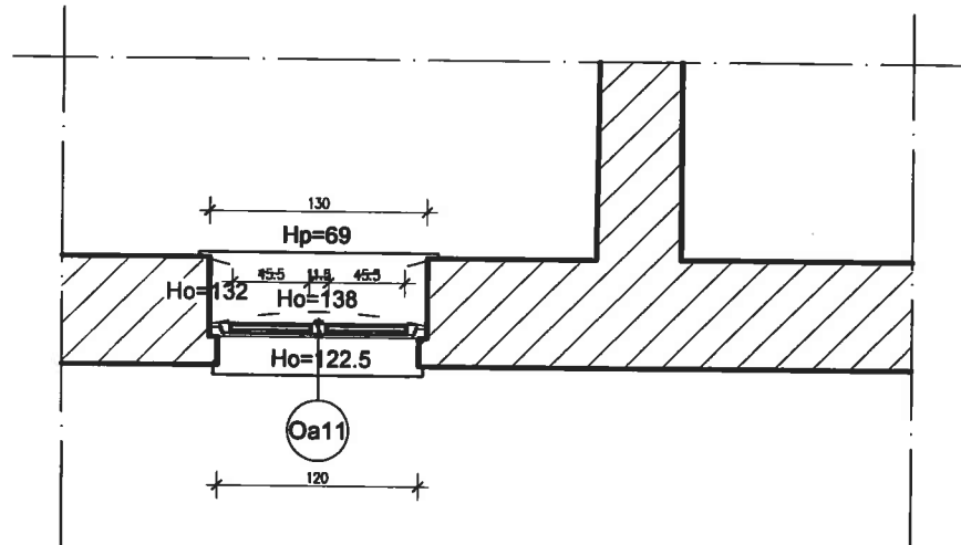
II PIĘTRO SKALA 1:50
