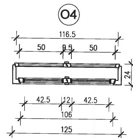
PRZYZIEMIE SKALA 1:25
