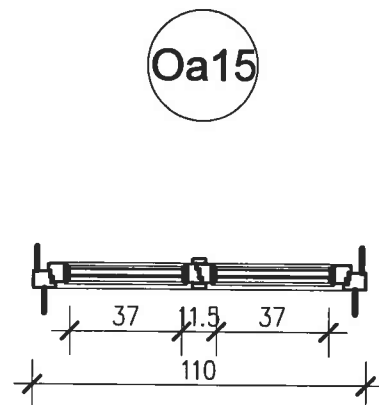
PODDASZE SKALA 1:25
