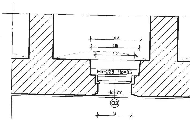
PRZYZIEMIA - INWENTARYZACJA SKALA 1:50
