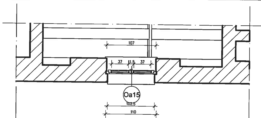
PODDASZE SKALA 1:50
