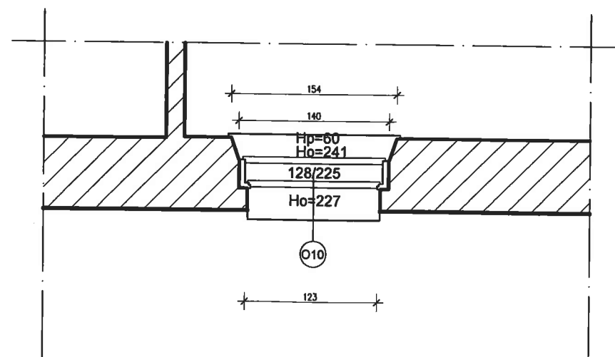
II PIĘTRO - INWENTARYZACJA SKALA 1:50
