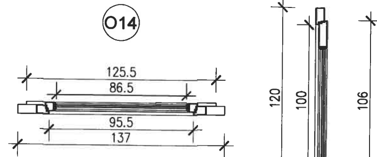
PODDASZE SKALA 1:25
