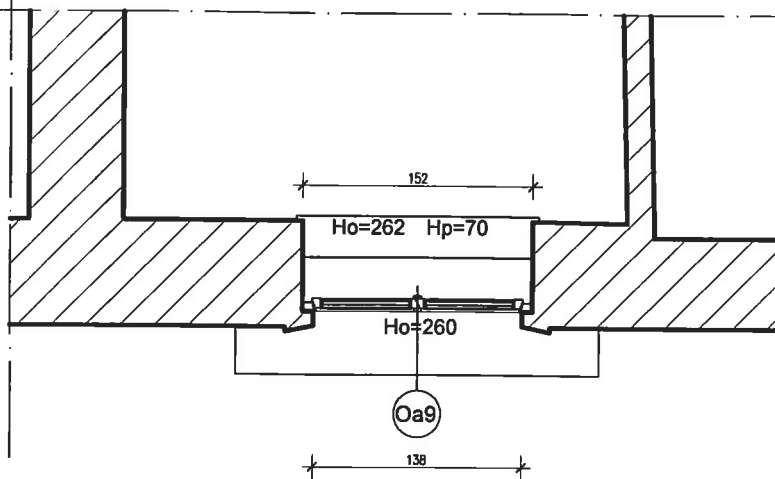
I PIĘTRO SKALA 1:50
