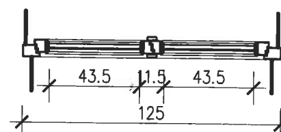
PRZYZIEMIE SKALA 1:25
