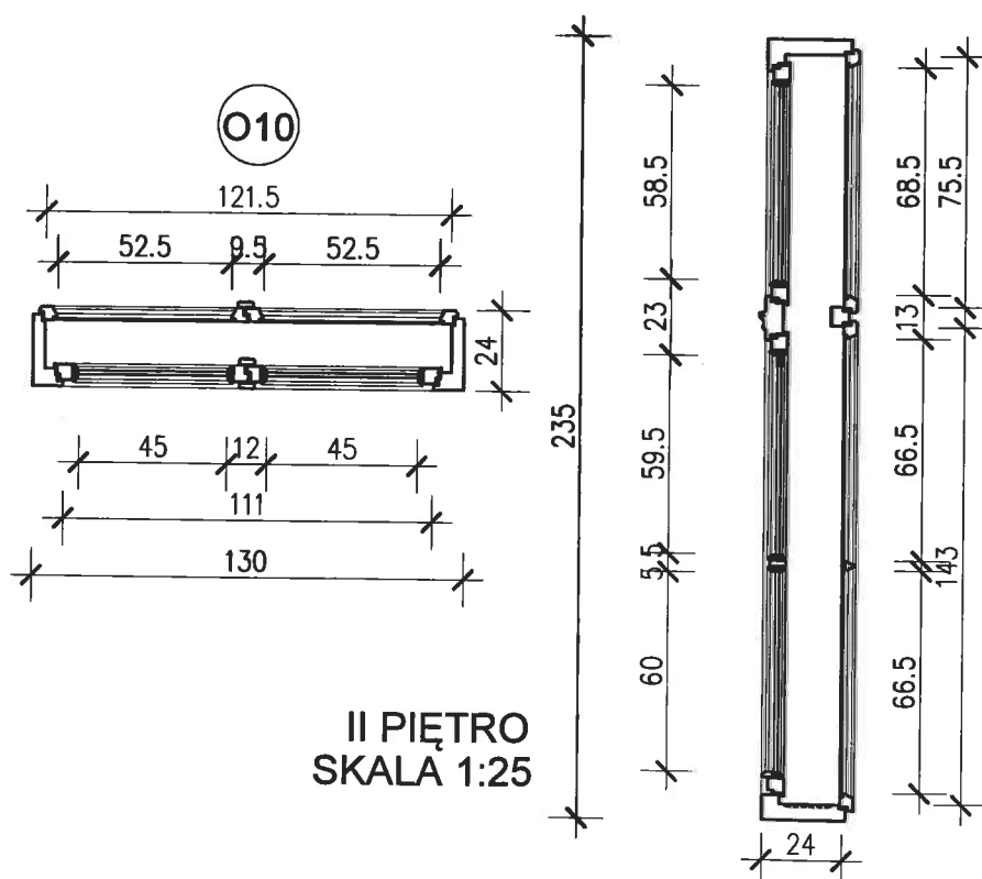
II PIĘTRO SKALA 1:25
