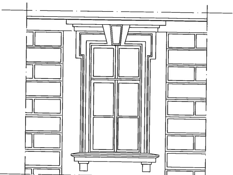
PARTER SKALA 1:50
