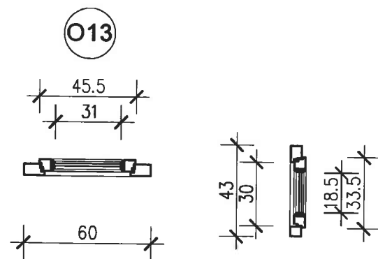
PODDASZE SKALA 1:25
