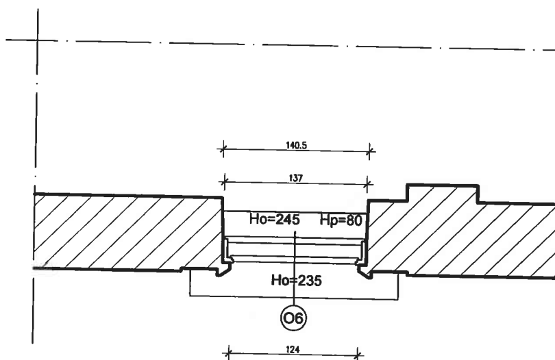
PARTER - INWENTARYZACJA SKALA 1:50
