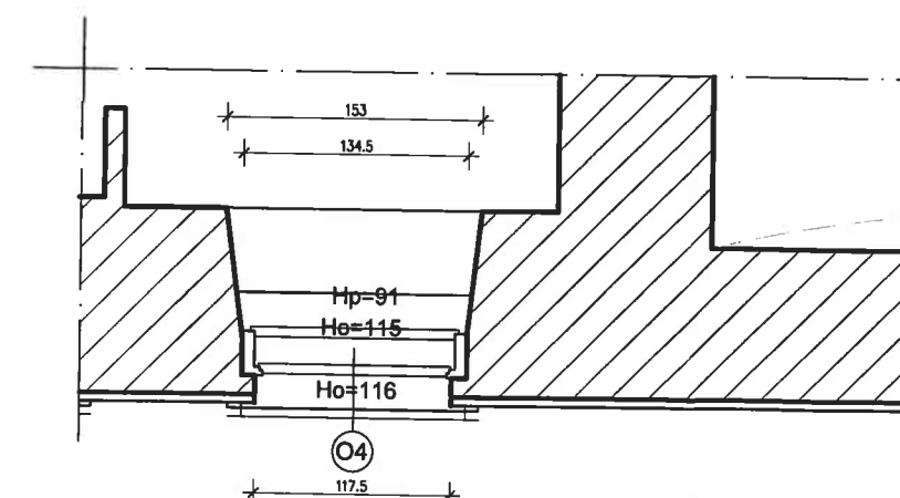
PRZYZIEMIE - INWENTARYZACJA SKALA 1:50
