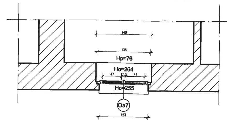
I PIĘTRO SKALA 1:50
