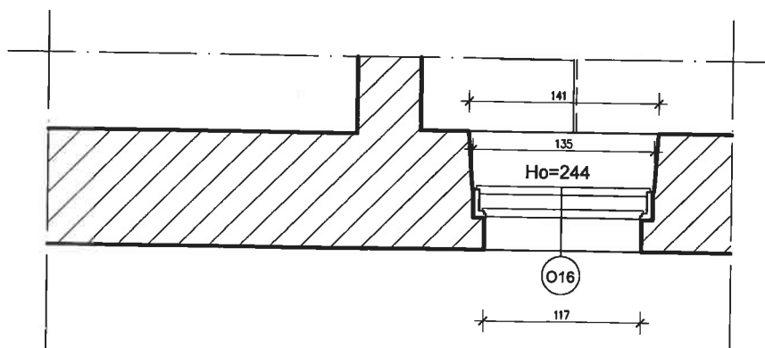
PARTER - INWENTARYZACJA SKALA 1:50
