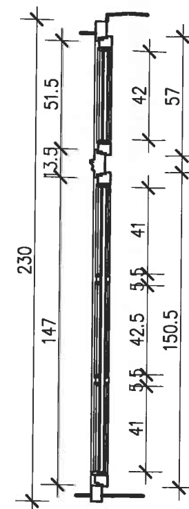
PARTER SKALA 1:25
