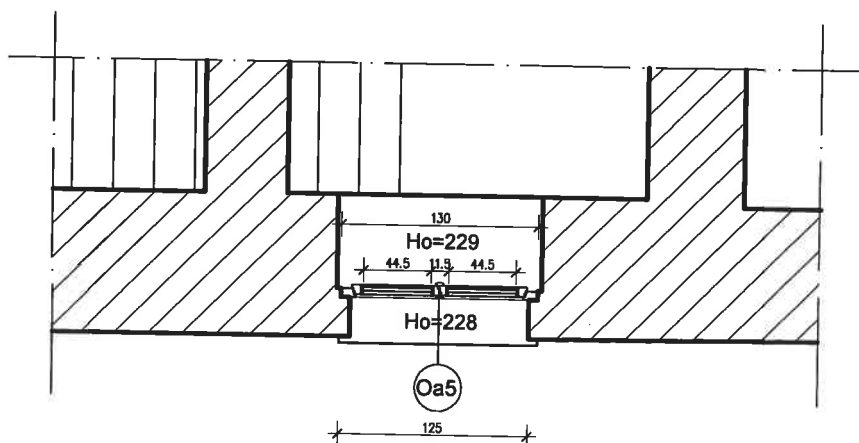
PARTER SKALA 1:50
