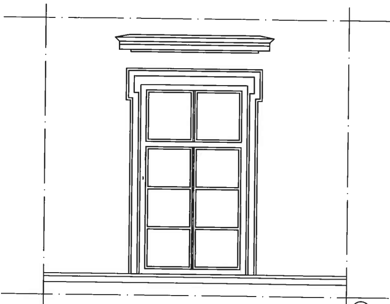
I PIĘTRO SKALA 1:50
