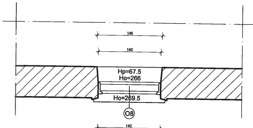
I PIĘTRO - INWENTARYZACJA SKALA 1:50
