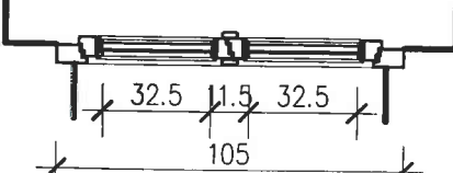
PRZYZIEMIE SKALA 1:25
