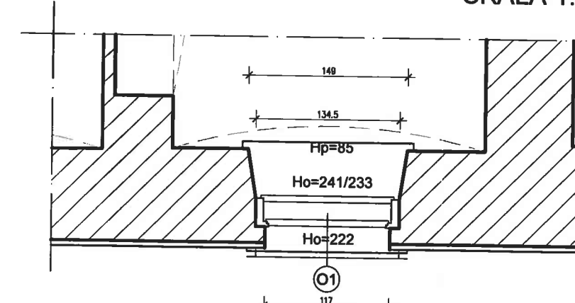
PRZYZIEMIE - INWENTARYZACJA SKALA 1:50
