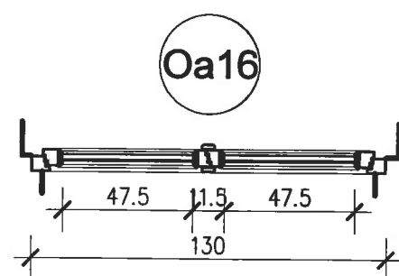
II PIĘTRO SKALA 1:25
