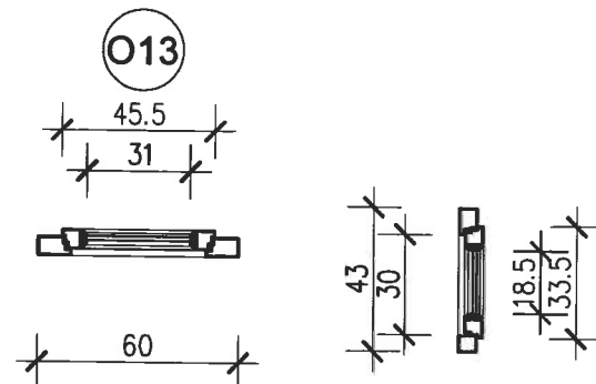
PODDASZE SKALA 1:25
