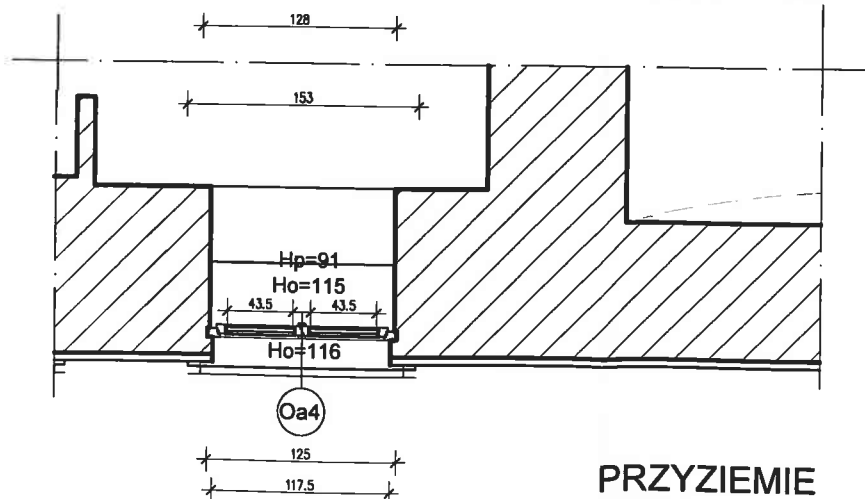
PRZYZIEMIE SKALA 1:50
