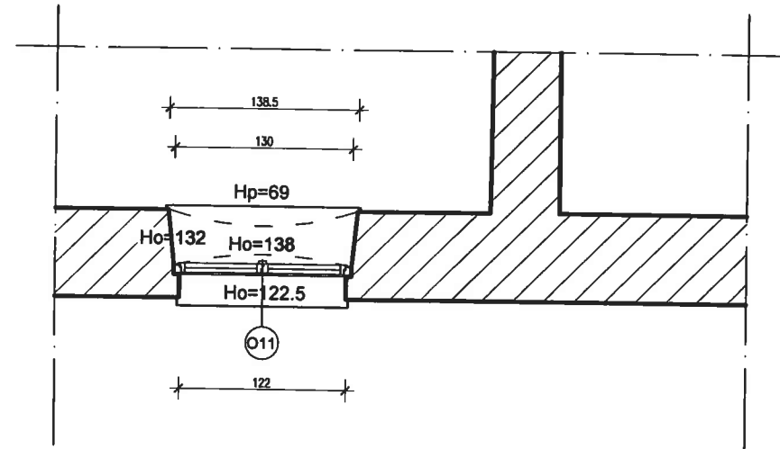
II PIĘTRO - INWENTARYZACJA SKALA 1:50
