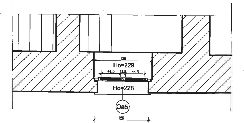
PARTER SKALA 1:50
