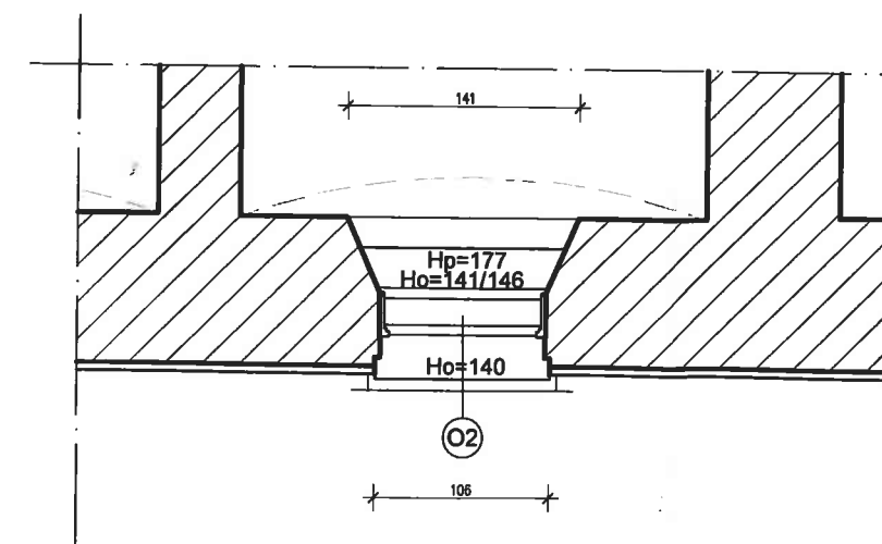
PRZYZIEMIE - INWENTARYZACJA SKALA 1:50
