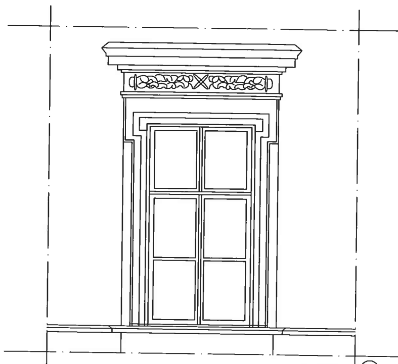
I PIĘTRO SKALA 1:50
