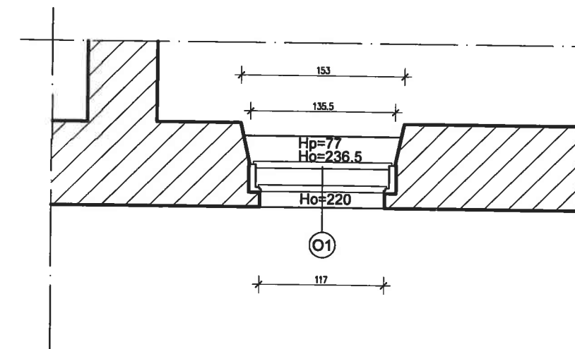
PARTER - INWENTARYZACJA SKALA 1:50
