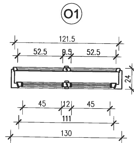
PARTER SKALA 1:25
