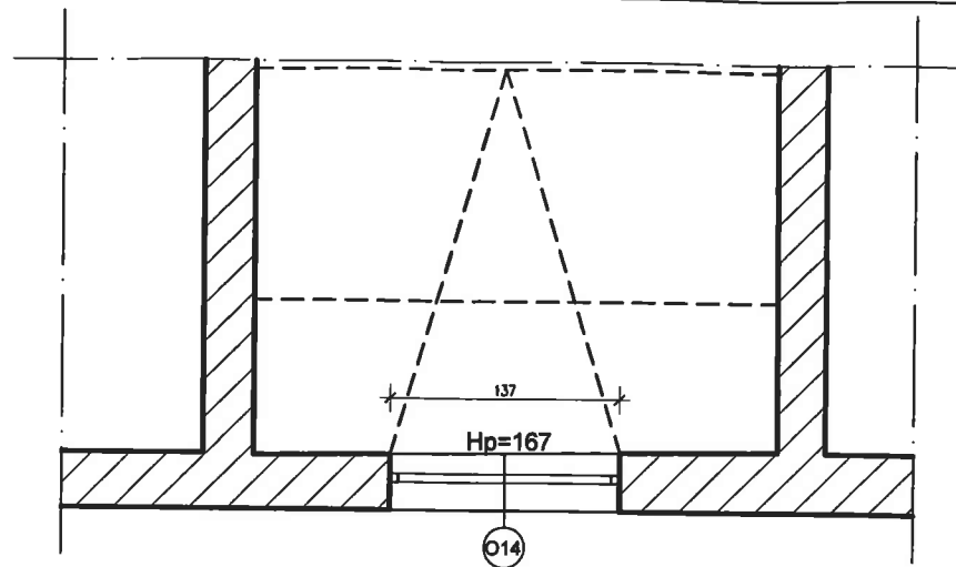
PODDASZE- INWENTARYZACJA SKALA 1:50
