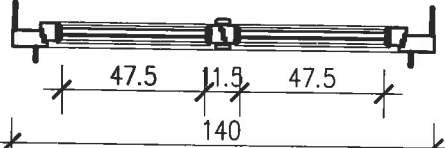
PARTER SKALA 1:25
