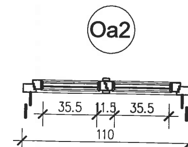
PRZYZIEMIE SKALA 1:25
