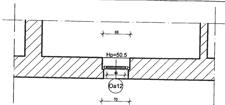
PODDASZE SKALA 1:50
