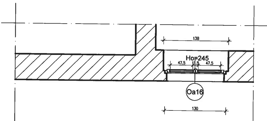
II PIĘTRO SKALA 1:50
