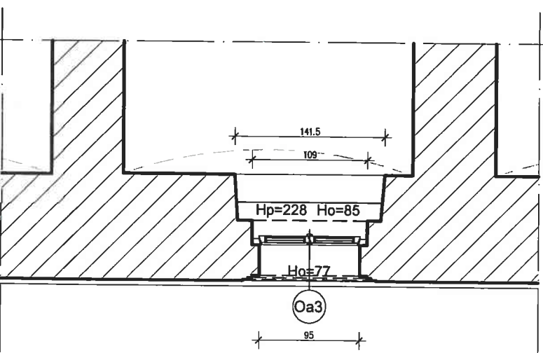
PRZYZIEMIE SKALA 1:50
