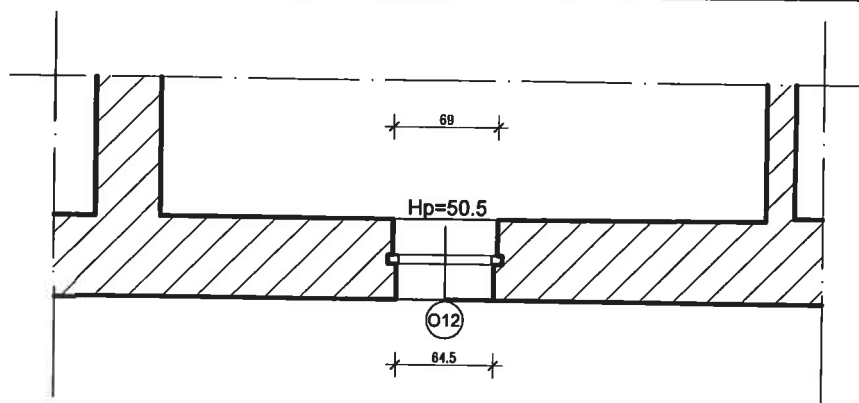
PODDASZE - INWENTARYZACJA SKALA 1:50
