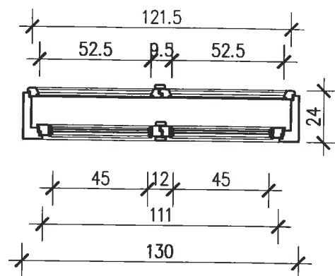
PIĘTRO SKALA 1:25
