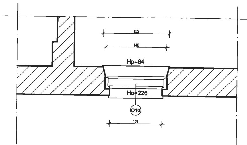
II PIĘTRO - INWENTARYZACJA SKALA 1:50
