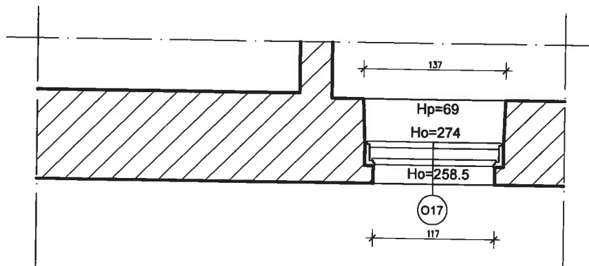
PIĘTRO - INWENTARYZACJA SKALA 1:50
