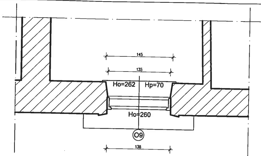
I PIĘTRO - INWENTARYZACJA SKALA 1:50
