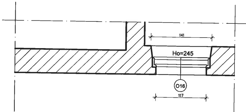
II PIĘTRO - INWENTARYZACJA SKALA 1:50
