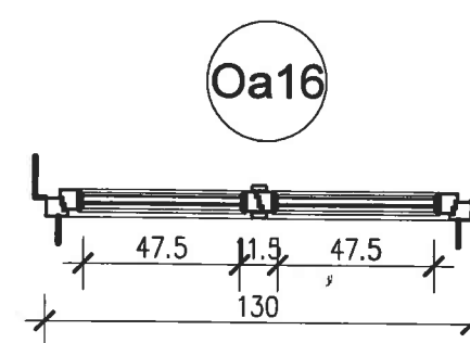
PARTER SKALA 1:25
