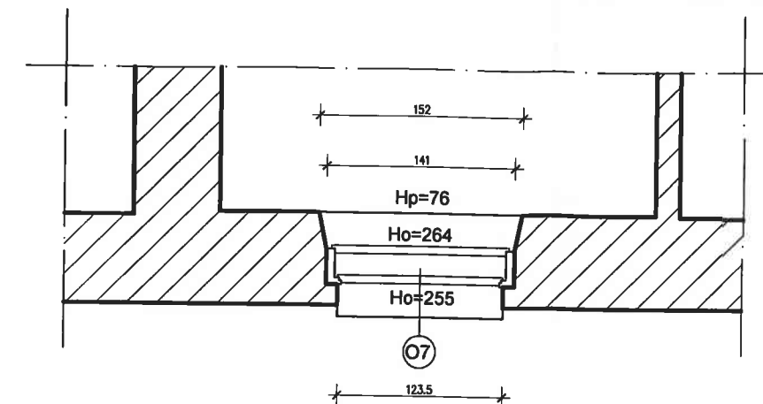
I PIĘTRO - INWENTARYZACJA SKALA 1:50
