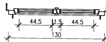
PARTER SKALA 1:25
