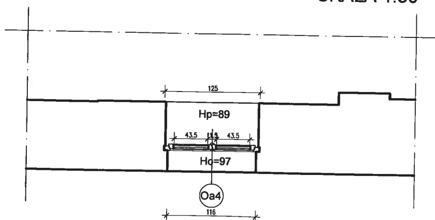
PRZYZIEMIE SKALA 1:50
