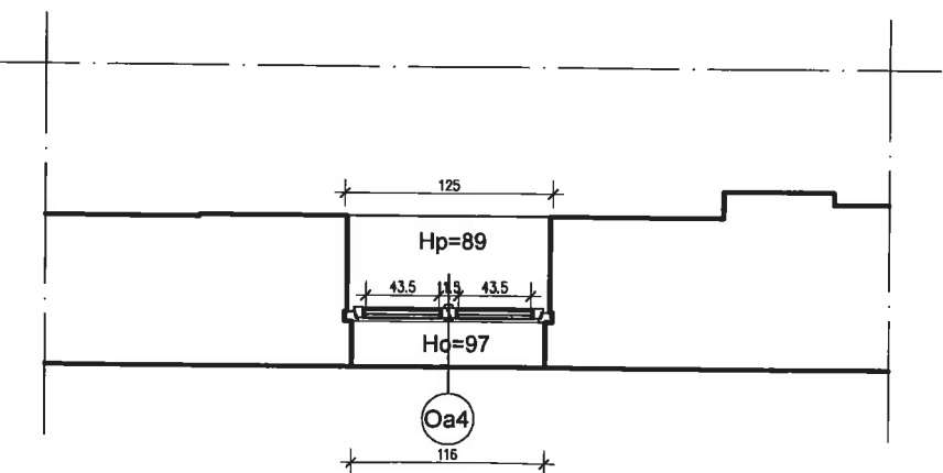
PRZYZIEMIE SKALA 1:50
