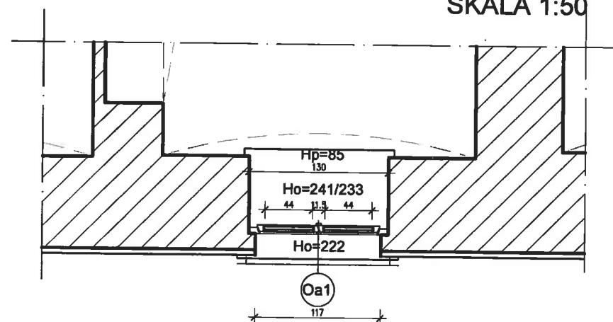
PRZYZIEMIE SKALA 1:50
