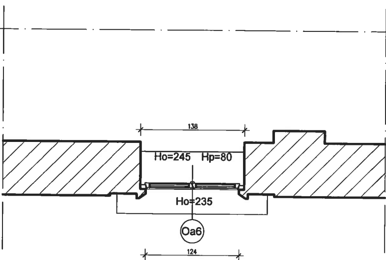
PARTER SKALA 1:50
