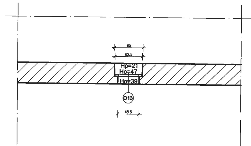
PODDASZE - INWENTARYZACJA SKALA 1:50
