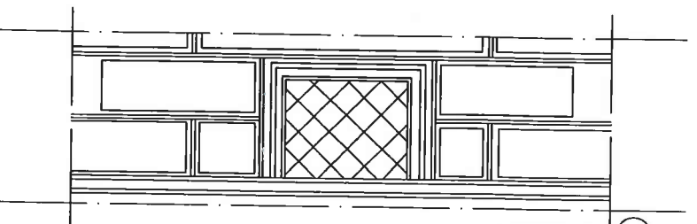
PRZYZIEMIE SKALA 1:50
