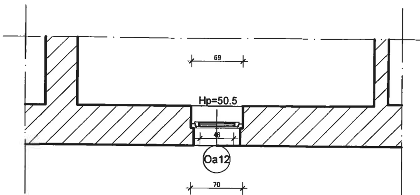
PODDASZE SKALA 1:50
