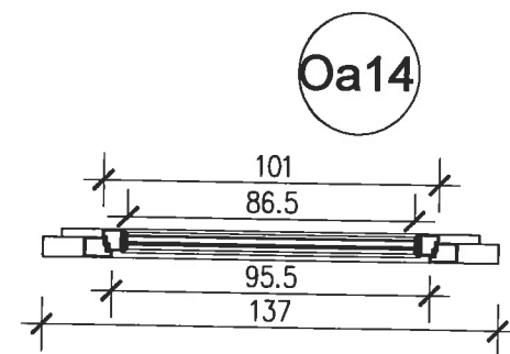
PODDASZE SKALA 1:25
